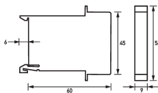
Dibujo acotado Vista de grupos
