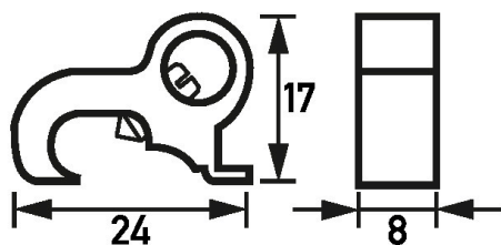
Dibujo acotado Bloqueos contra reconexiones RH-SPE
