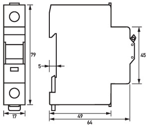
Dibujo acotado Interruptores-seccionadores RH 032-100
