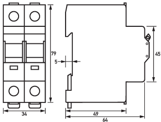
Dibujo acotado Interruptores-seccionadores RH 032-200
