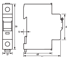
Dibujo acotado Vista de grupos
