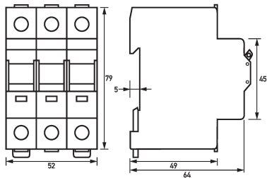
Dibujo acotado Interruptores-seccionadores RH 032-300
