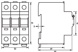
Maßzeichnung Gruppenansicht
