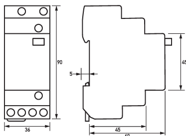
Dibujo acotado Interruptores de impulsos (interruptores remotos) RS 024-002
