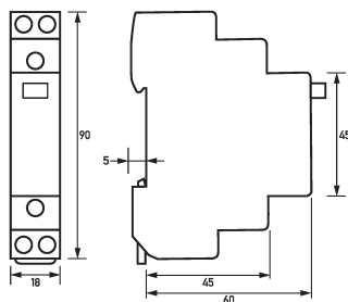
Dibujo acotado Interruptores de impulsos (interruptores remotos) RS 024-110
