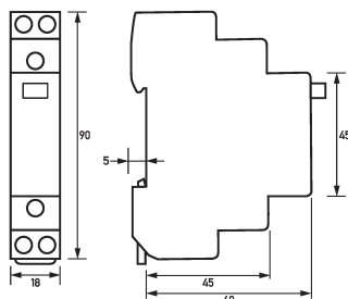
Dibujo acotado Interruptores de impulsos (interruptores remotos) RS 024-200
