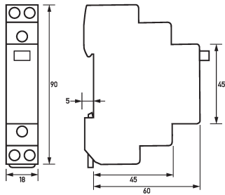
Dibujo acotado Relés de instalación RI 008-110
