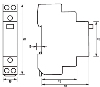
Dibujo acotado Relés de instalación RI
