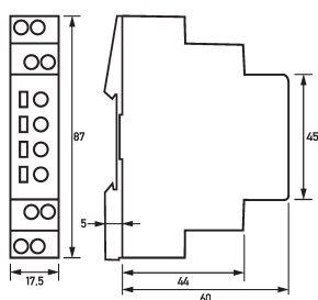
Maßzeichnung Zeitrelais RZQ 248
