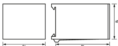
Maßzeichnung Sicherungssteckersätze DSE Do-50
