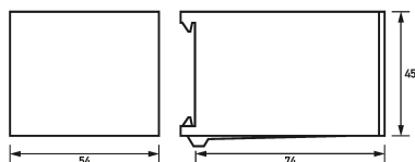
Maßzeichnung Sicherungssteckersätze DSE Do-40
