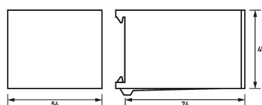
Dibujo acotado Juegos de conectores de fusibles DSE Do-32
