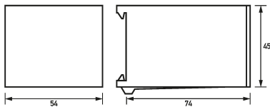
Dibujo acotado Juegos de conectores de fusibles DSE Do-13
