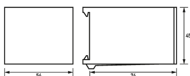
Dibujo acotado Juegos de conectores de fusibles DSE Do-01
