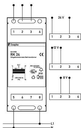
Ejemplo de cableado Transformadores de timbre RK 24
