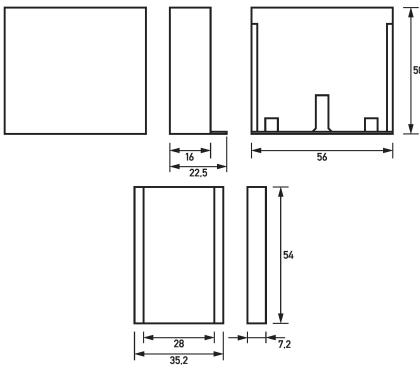
Dibujo acotado Juegos de montaje RK M54
