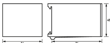
Maßzeichnung Sicherungssteckersätze DSE Do2-40 MI
