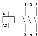
Ejemplo de cableado Contactores de instalación HS 2-230AC/25-30
