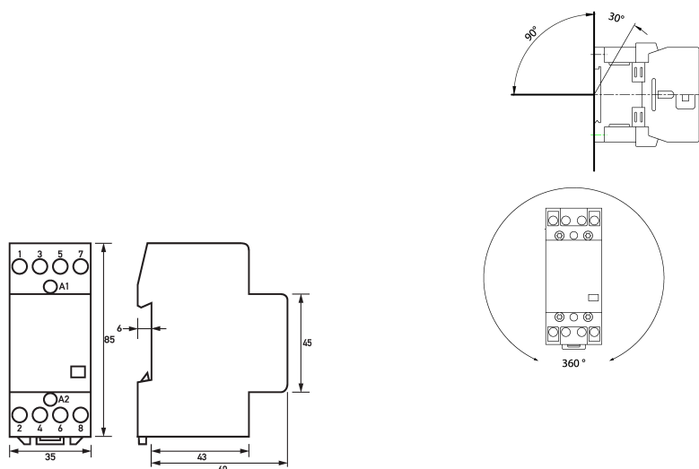
Dibujo acotado Contactores de instalación HS 2-230AC/25-30
