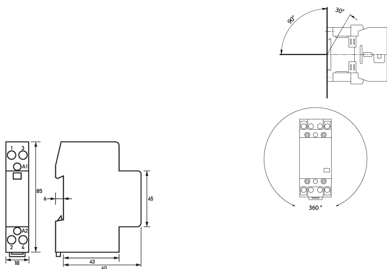
Dibujo acotado Contactores de instalación HS 1-230AC/20-10
