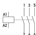
Schaltungsbeispiel Installationsschütze HS 3-230AC/63-30
