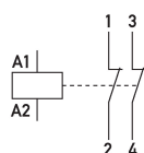
Ejemplo de cableado Contactores de instalación HS 3-230AC/40-02
