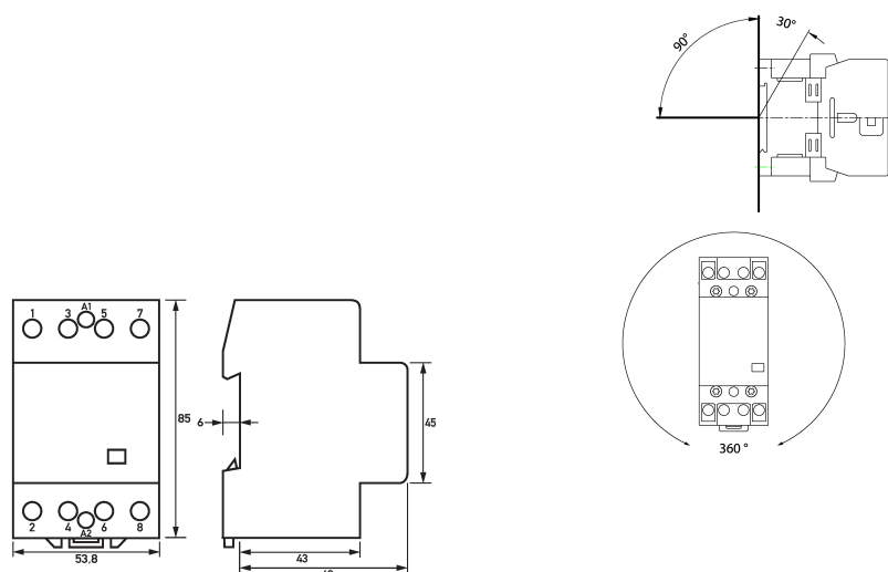
Maßzeichnung Installationsschütze HS 3-230AC/40-40
