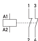
Ejemplo de cableado Contactores de instalación HS 1-230AC/20-02
