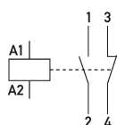
Ejemplo de cableado Contactores de instalación HS 1-230AC/20-11
