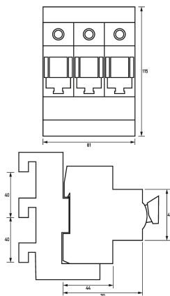
Dibujo acotado Vista de grupos
