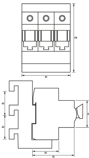
Maßzeichnung Sicherungslasttrennschalter Tytan II Do-63-3/B
