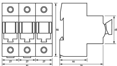
Maßzeichnung Sicherungslasttrennschalter Tytan
