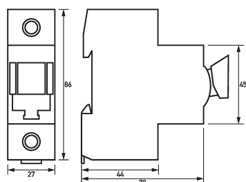
Maßzeichnung Sicherungslasttrennschalter Tytan
