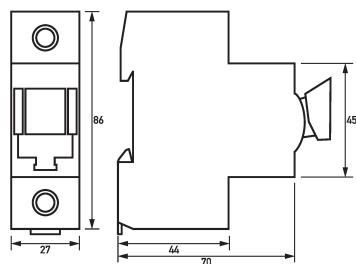
Maßzeichnung Sicherungslasttrennschalter Tytan II Do-04-1/S
