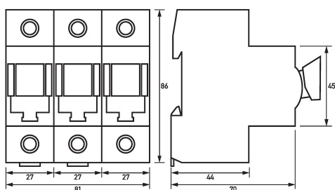
Maßzeichnung Sicherungslasttrennschalter Tytan II Do-35-3/S
