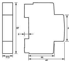
Dibujo acotado Vista de grupos
