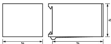
Dibujo acotado Juegos de conectores de fusibles DSE Do2-02 EI
