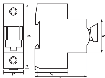
Maßzeichnung Sicherungslasttrennschalter Tytan II Do-63-1
