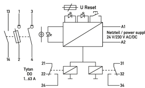
Anschlussschema
