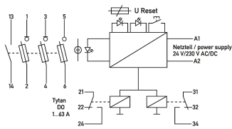
Esquema de conexiones
