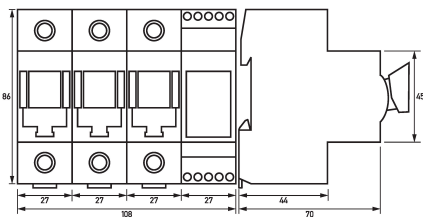
Maßzeichnung Gruppenansicht
