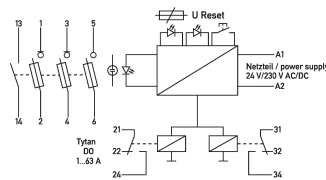
Anschlussschema
