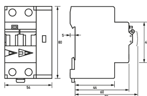
Maßzeichnung Fehlerlichtbogen-Schutzeinrichtungen DAFDD 1 C40/0,03/2-A KV
