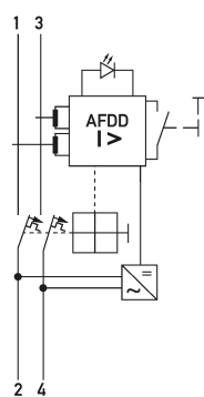
Schaltungsbeispiel Fehlerlichtbogen-Schutzeinrichtungen DAFDD 1 C40/0,03/2-A KV
