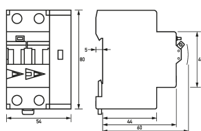
Maßzeichnung Fehlerlichtbogen-Schutzeinrichtungen DAFDD 1 C10/0,03/2-A KV
