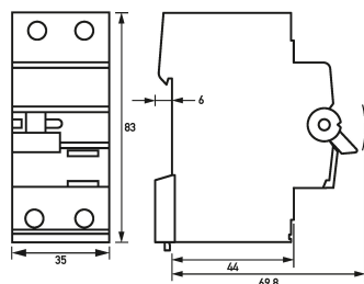
Dibujo acotado Combinaciones de interruptores diferenciales e interruptores magnetotérmicos RCBO 2 C15/0,03/2-A
