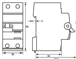
Maßzeichnung Gruppenansicht
