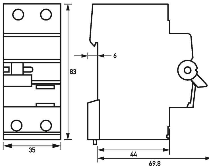
Maßzeichnung RCBO 2, Typ A, 2-polig (Gruppenansicht)
