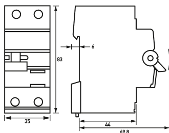
Maßzeichnung Gruppenansicht
