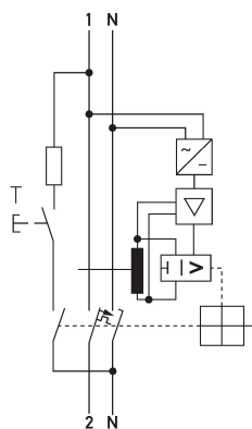
Esquema de conexiones DRCBO 4 HP, 1 polos + N
