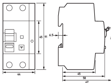
Dibujo acotado Vista de grupos
