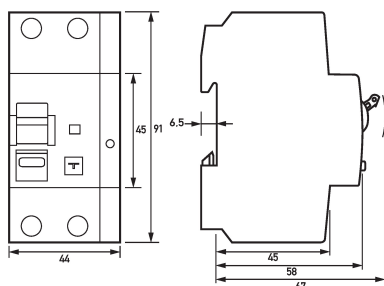
Maßzeichnung FI-/LS-Kombinationen DRCBO 4 C16/0,10/1N-PV
