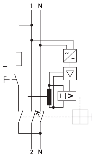
Anschlussschema DRCBO 4 Typ B+, 1+N-polig
